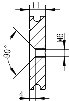
A-A 1 : 1.5
